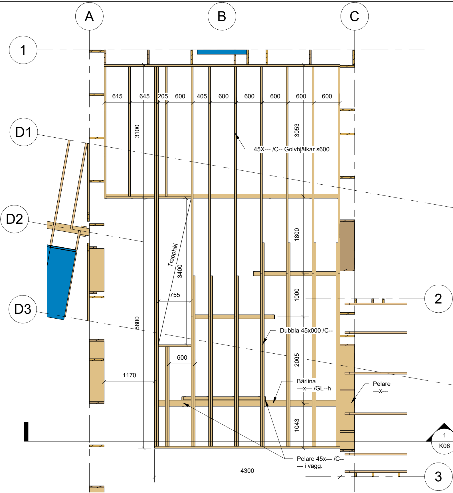
1 Bjälklagsplan 1 : 50
