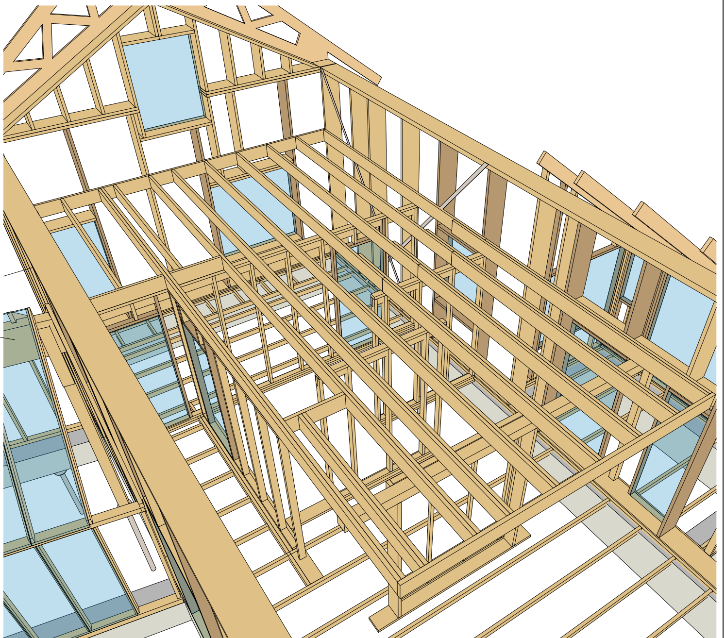
2 Översikt bjälklag
