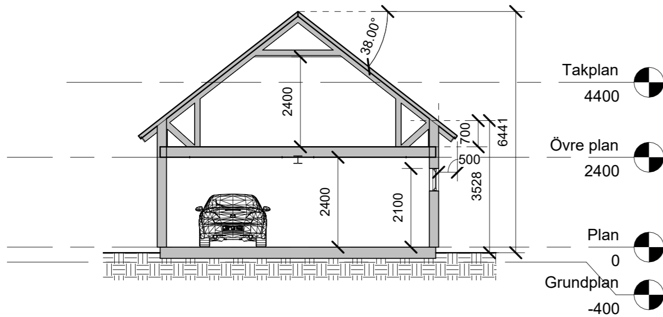
1 Sektion A-A 1 : 100
