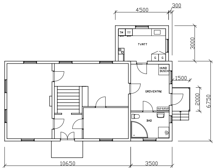
BOTTENPLAN 1:100
