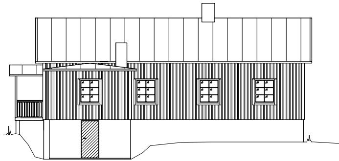
FASAD MOT NØRØ 1:100
