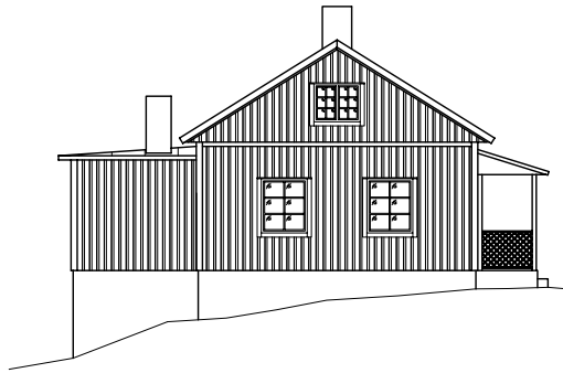
FASAD MOT VÆSTER 1:100
