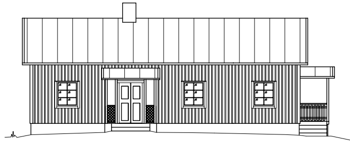
FASAD MOT SØDER 1:100
