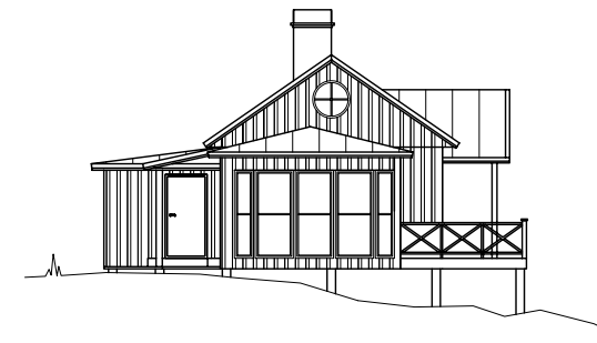
BOSTADSHUS FASAD MOT VÄSTER 1:100
