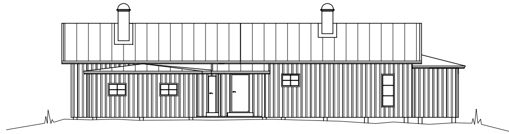
BOSTADSHUS FASAD MOT NORR 1:100
