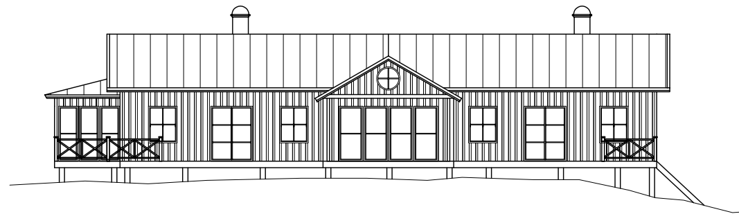
BOSTADSHUS FASAD MOT SÖDER 1:100
