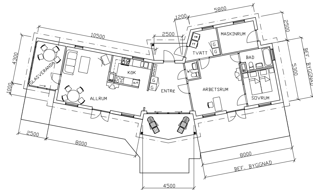
BOSTADSHUS PLAN 1:100
